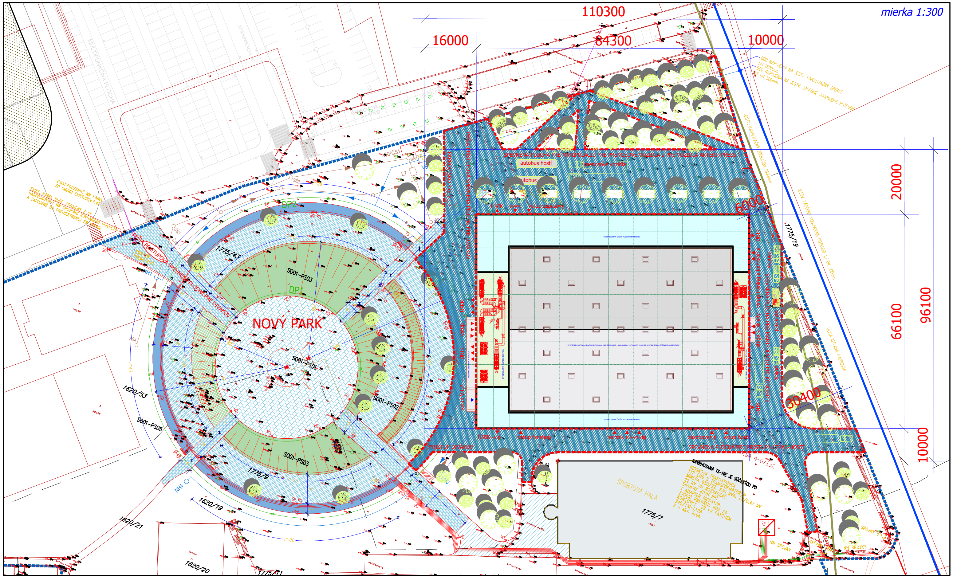
SITUÁCIA OSADENIA NOVEJ MULTIFUNKČNEJ ŠPORTOVEJ HALY S PREPOJENÍM NA NOVÉ NÁMESTIE A NA OSTATNÉ KOMUNIKÁCIE MESTA
